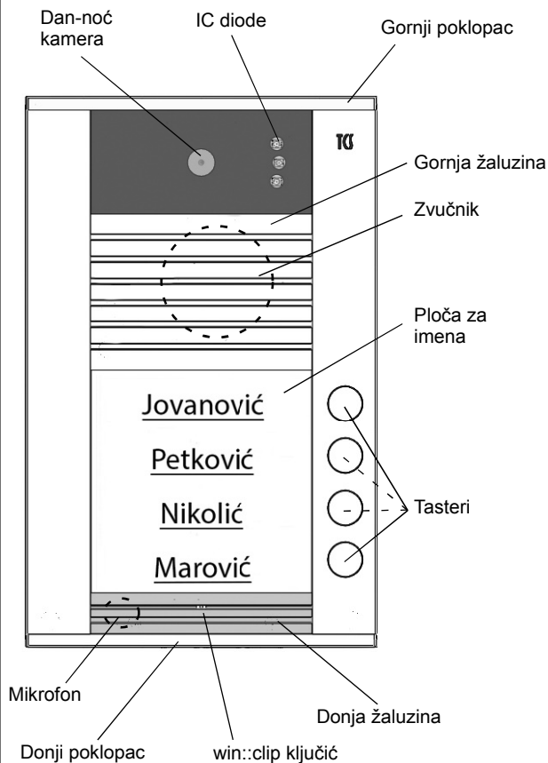
SI. 1 Pozivna stanica pogled sa prednje strane
